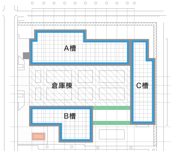
配置図
