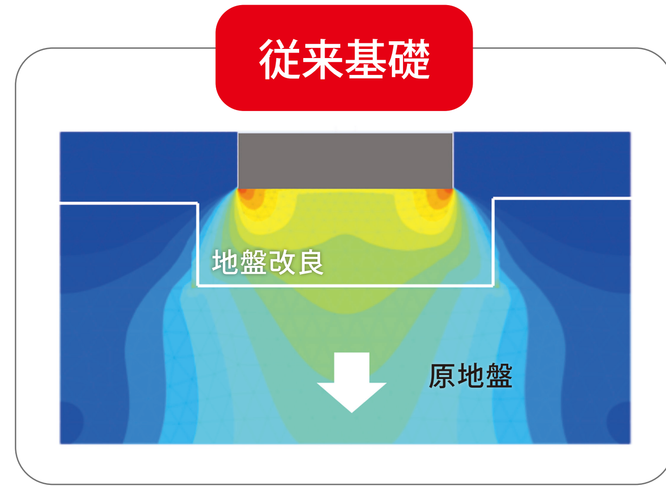
FEM による応力の比較
