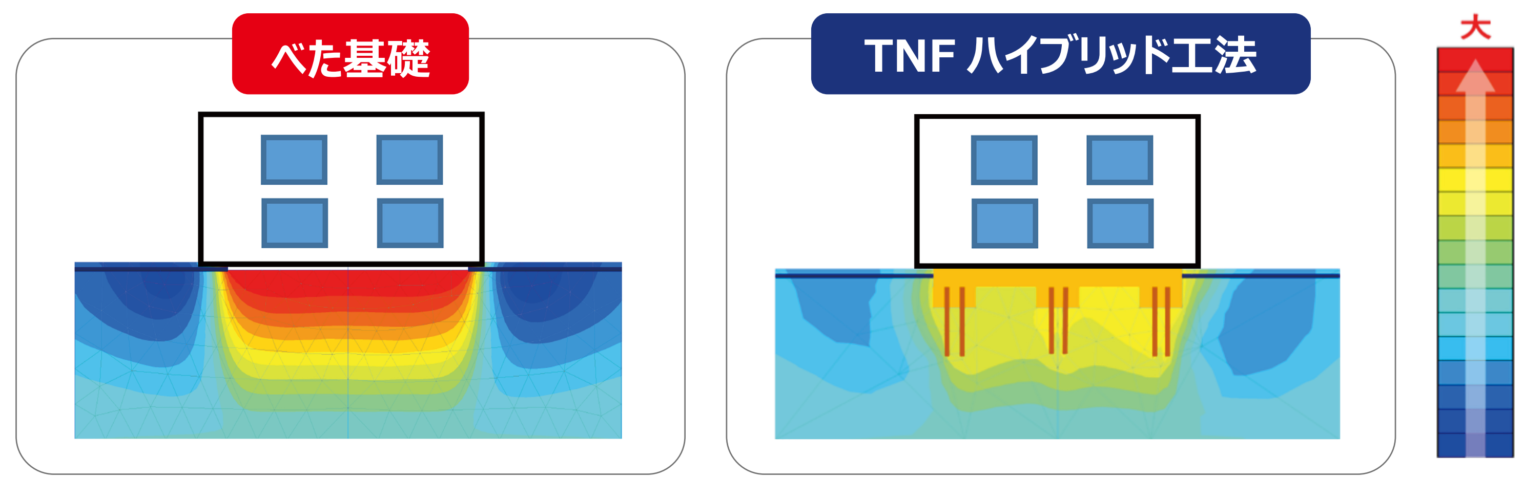
FEM による液状化解析 (沈下量の比較)
